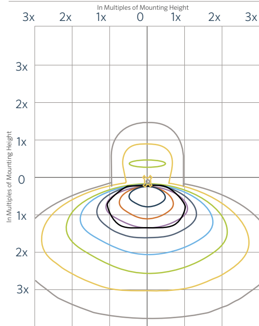
A-BR10 L20 GV Isofootcandle Plot
