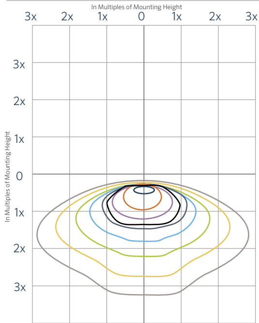
A-BR10 L13 GP Isofootcandle Plot
