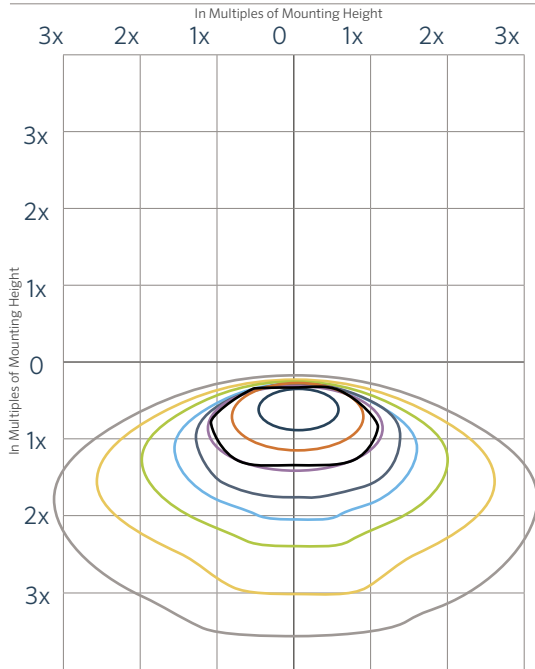
A-BR10 L20 GP Isofootcandle Plot
