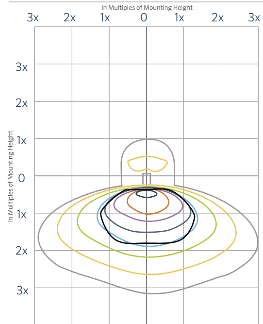
A-BR10 L13 GV Isofootcandle Plot
